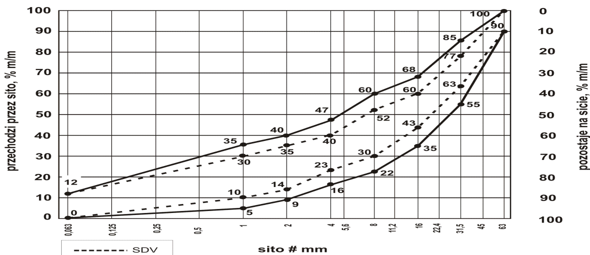
Rys. 10. Uziarnienie mieszanki niezwiązanej 0/63 dla podbudowy pomocniczej Aby zapewnić jednorodność i ciągłość uziarnienia mieszanki, oprócz wymagań podanych na rysunkach 8 - 10, 90% uziarnień zbadanych w ramach Zakładowej Kontroli Produkcji (ZKP) w okresie do 6 miesięcy powinno spełniać wymagania podane w Tabelcy 2 i 3.
