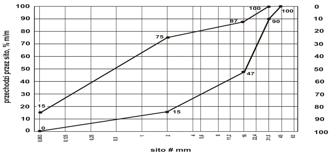
Rys. 5. Uziarnienie mieszanki niezwiązanej 0/31,5 dla warstwy mrozoochronnej
