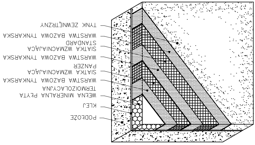
WZMOCNIENIE DODATKOWE
