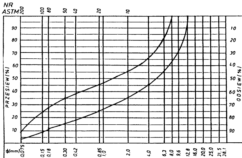
Rys.6. Krzywe graniczne uziarnienia mieszanki mineralnej 0+12,8 mm do warstwy wiążącej, wyrównawczej i wzmacniającej z betonu asfaltowego dla KR 1-2
