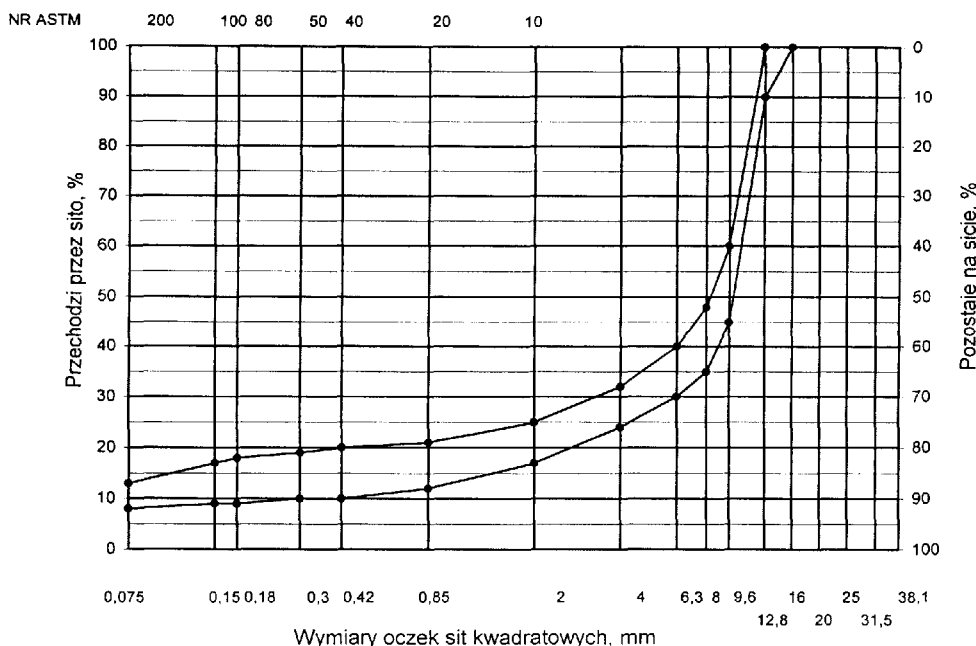
Rys. 5. Krzywe graniczne uziarnienia mieszanki mineralnej SMA od 0 do 12,8 mm do warstwy ścieralnej.
