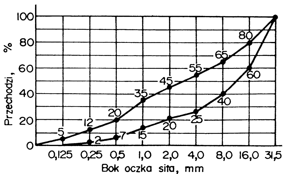
Rysunek 1. Graniczne krzywe uziarnienia do betonu C25/30 B 30 od 0 do 31,5 mm.
