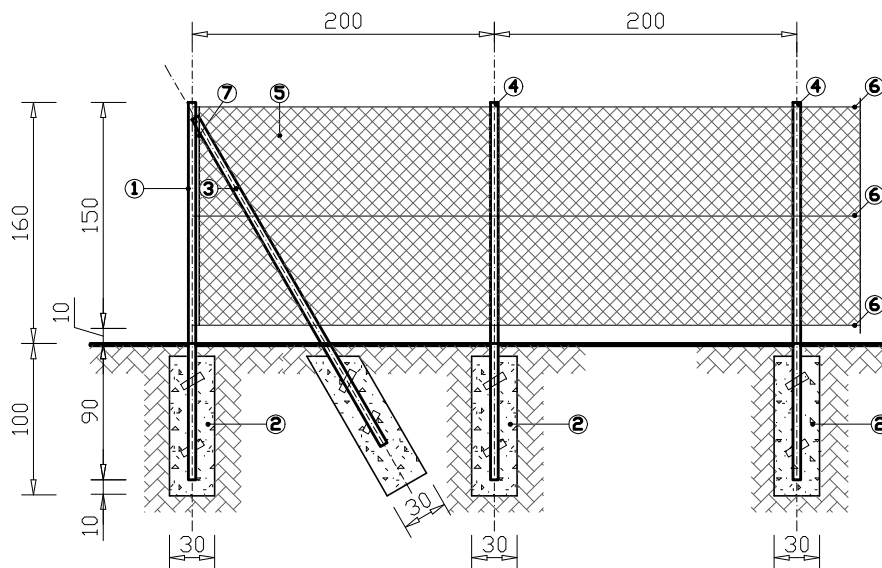
SŁUP SKRAJNY/NAROŻNY
