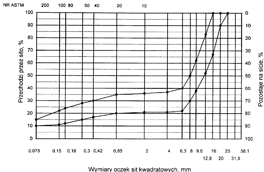
Rys. 5. Krzywe graniczne uziarnienia mieszanki mineralnej BA od 0 do 20 mm (mieszanka o nieciąłym uziarnieniu) do warstwy ścieralnej nawierzchni drogi o obciążeniu ruchem od KR3 do KR6
