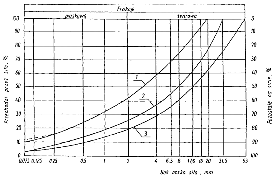
Rysunek 1. Pole dobrego uziarnienia kruszywa przeznaczonych na warstwy z kruszywa.
