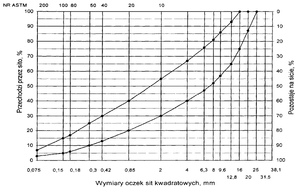
Rys. 1. Krzywe graniczne uziarnienia mieszanki mineralnej BA od 0 do 20 mm do warstwy wiążącej i wyrównawczej nawierzchni drogi o obciążeniu ruchem KR1 lub KR2
