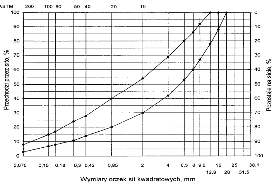
Rys. 2. Krzywe graniczne uziarnienia mieszanki mineralnej BA od 0 do 16 mm do warstwy wiążącej i wyrównawczej nawierzchni drogi o obciążeniu ruchem KR1 lub KR2
