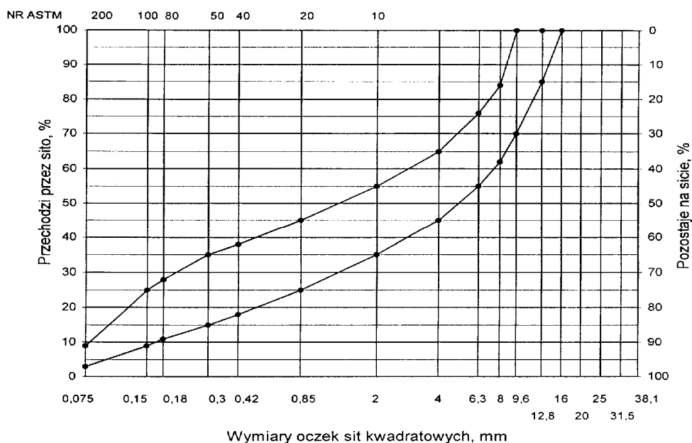
Rys. 3. Krzywe graniczne uziarnienia mieszanki mineralnej BA od 0 do 12,8 mm do warstwy wiążącej i wyrównawczej nawierzchni drogi o obciążeniu ruchem KR1 lub KR2
